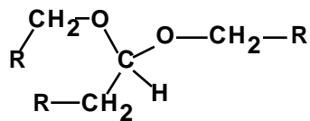
acetal
