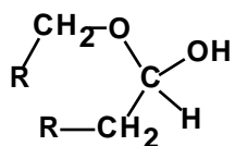
hemiacetal
